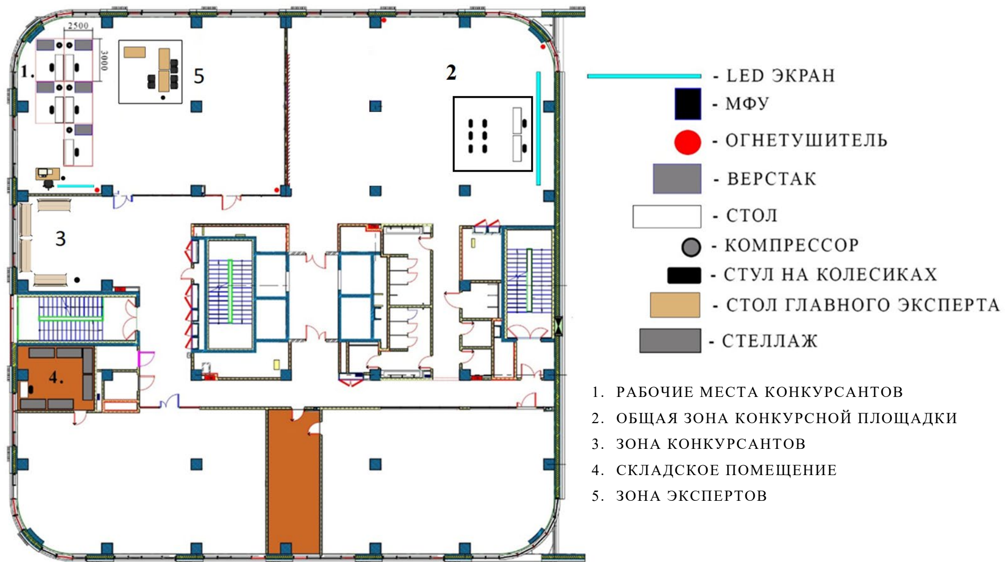
Рисунок 1 - План застройки площадки компетенции «Мехатроника»
