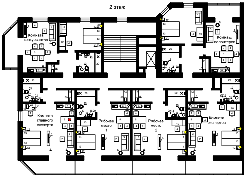
2 этаж
